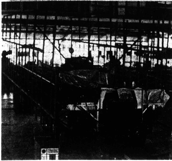
Poto antap i soim ol bun bilong wanpela bas, em ol i wokim long Port Moresby yet. Ol i baim ensin tasol wantaim bun bilong holim wil samting. Na haus bilong bas ol man bilong Moresby yet i wokim. Hia yu lukim ol bun tasol bilong bas ol i weldim na sodaim. Na ol windo na sia na kapa bai ol i baim na wokim long Moresby.
